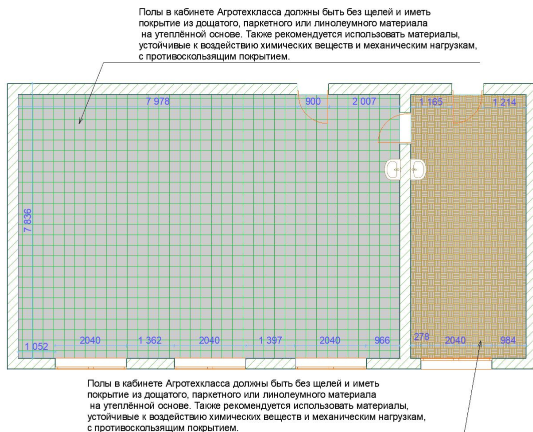
План полов
