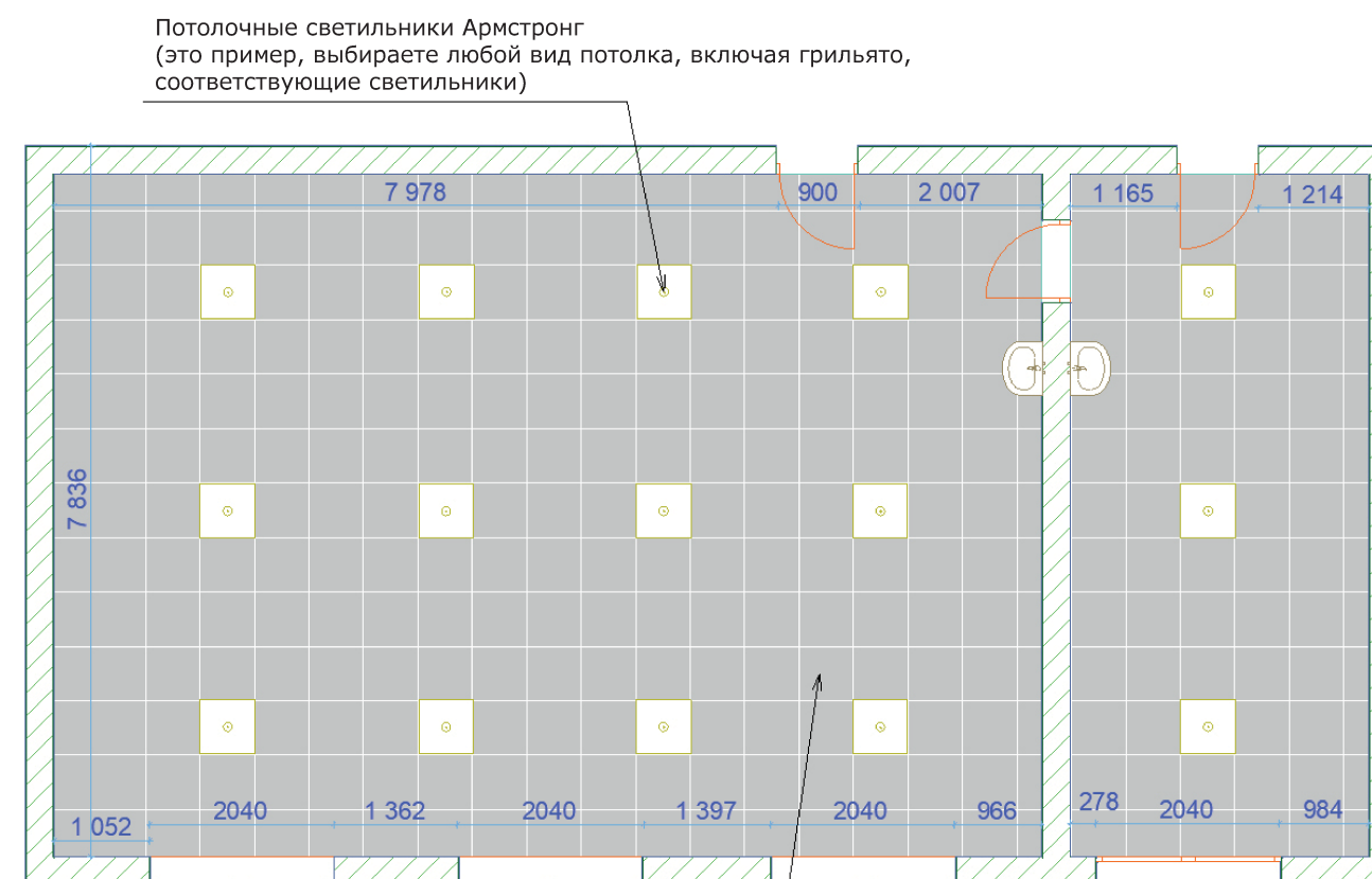
План потолков
